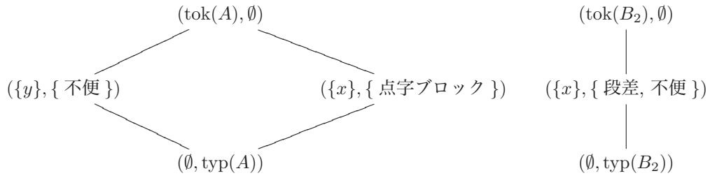
図 1: 分類 A の形式概念束のハッセ図 (左) と, 分類 B_2 の形式概念束のハッセ図 (右)
