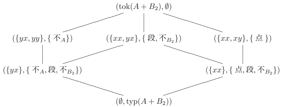
図 2: 分類 A + B_2 の形式概念束のハッセ図
