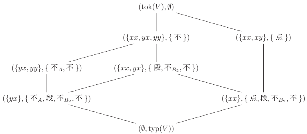
図 3: 分類 V の形式概念束のハッセ図
