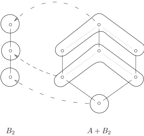
図 5: 分類 B_2 と A + B_2 の形式概念束の概念間の対応関係
