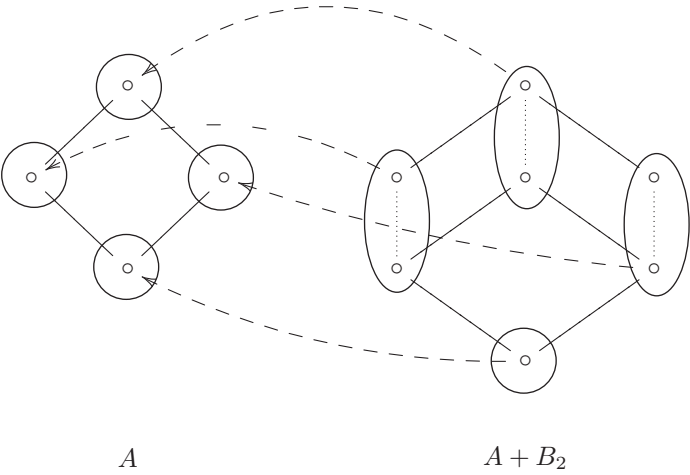
図 4: 分類 A と A + B_2 の形式概念束の概念間の対応関係
