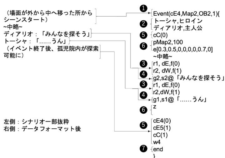
図.3.1.2-1.シナリオデータフォーマットの対応
