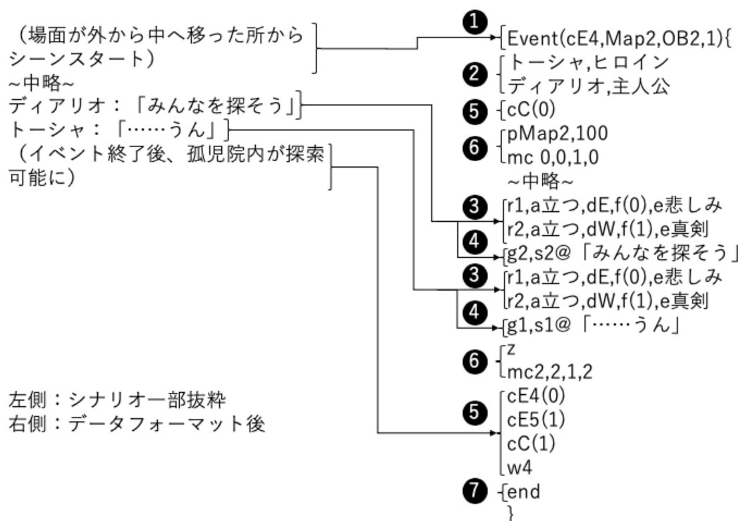
図 3.1.2-1 シナリオデータフォーマット
