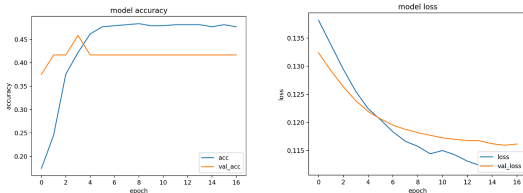
モデル3 (クロマグラム)
