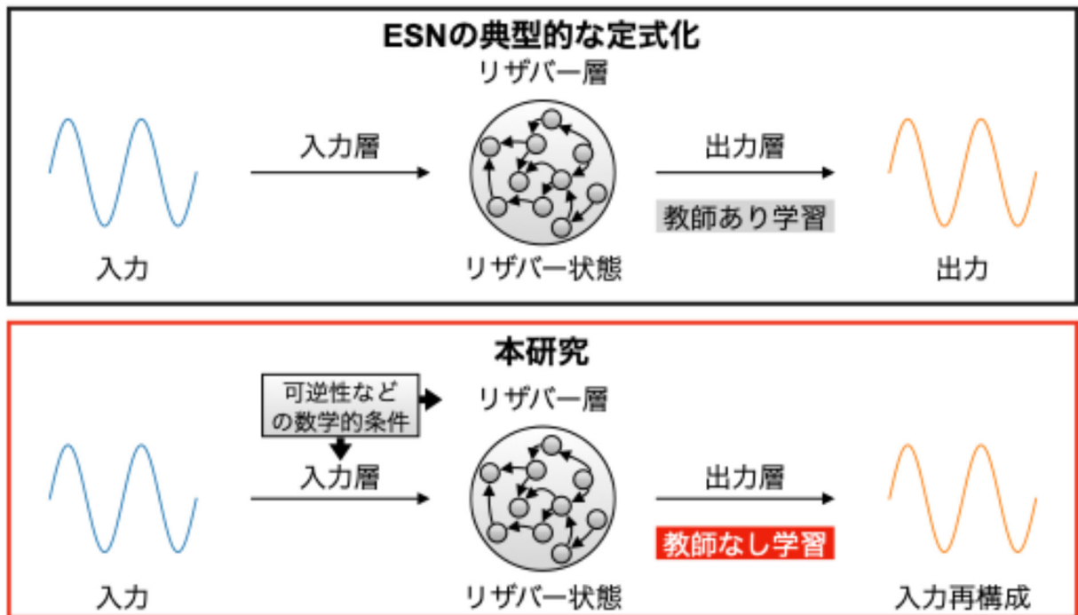
図1 ESNにおける入力再構成の定式化
