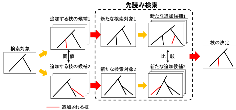
図4 先読み検索
