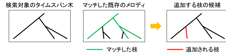
図6 枝の追加
